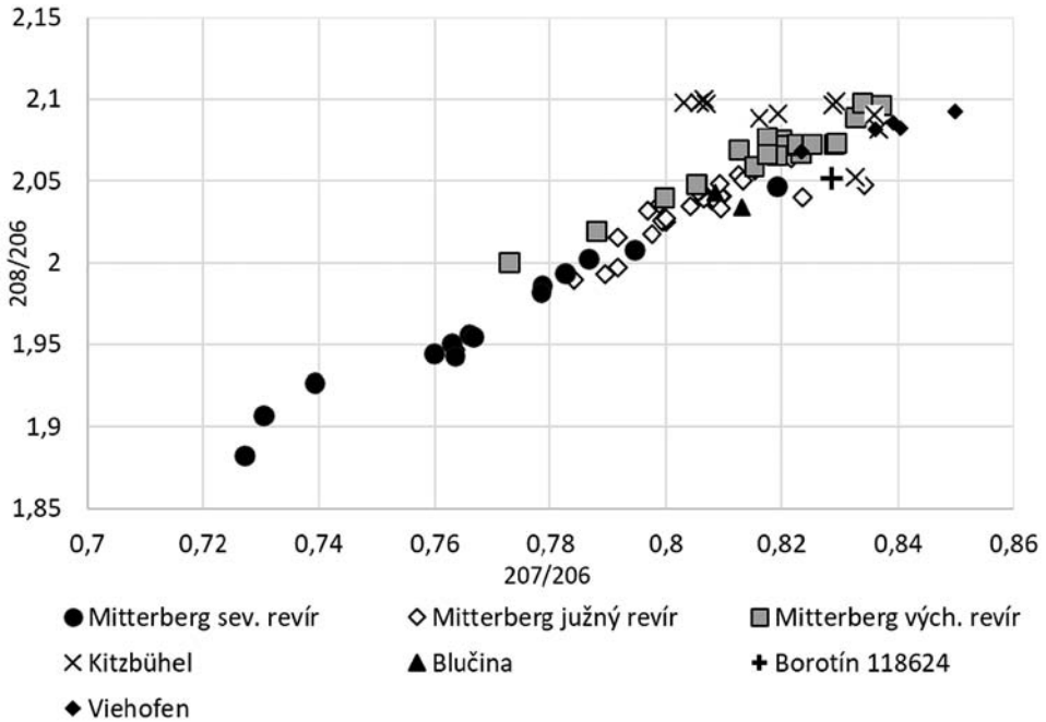
Obr. 4. Porovnanie stabilných izotopov olova jednotlivých regiónov vo Východných Alpách s hodnotami zliatkov z Blučiny 1 a Borotína. Podľa Pernicka – Lutz – Stöllner 2016 . Fig. 4. A comparison of the stable isotopes of lead from individual regions in the Eastern Alps with the values of ingots from Blučina 1 and Borotín. After Pernicka – Lutz – Stöllner 2016 .
